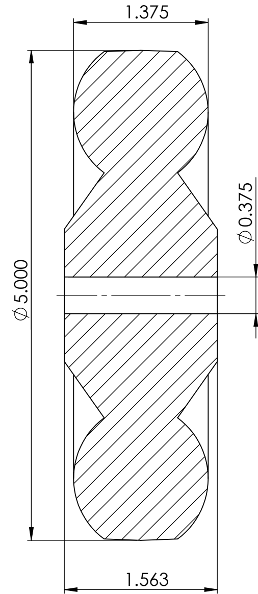
SECTION A-A SCALE 1 : 1
