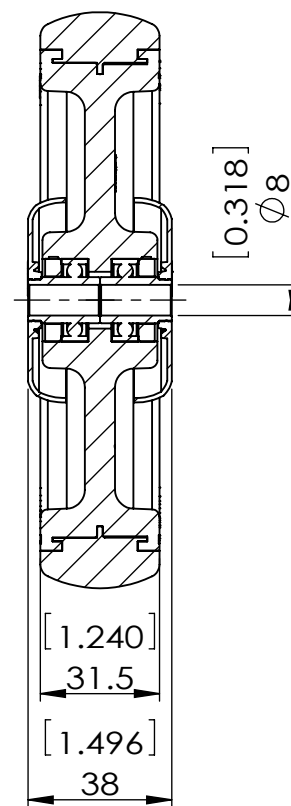
A-A (1 : 2)
