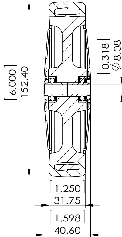
SECTION A-A
