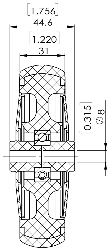
SECTION A-A
